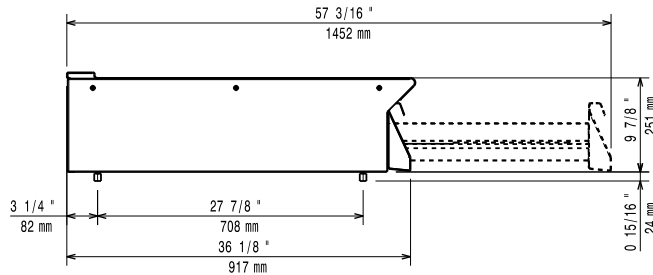
Boven aanzicht
